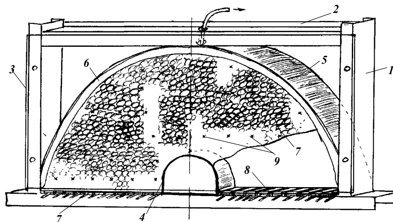
Рис. 2. Общий вид модели
