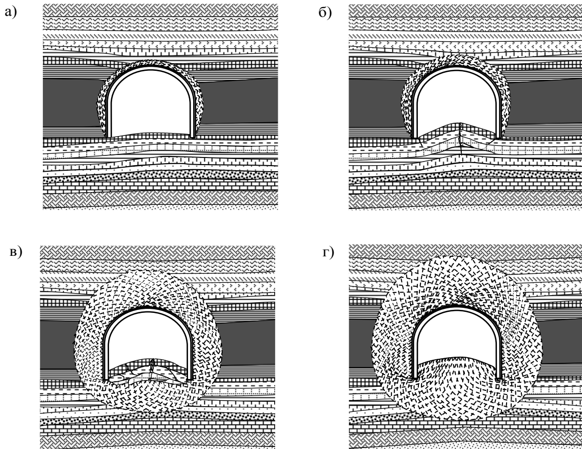
Рис. 1. Схемы механизма пучения почвы выработки на разных этапах ее существования: а, б - складкообразование породных слоев за счет формирования зоны разрушения вокруг выработки; в - выдавливание разрушенных пород в полость выработки под действием веса вышележащих пород, вмещающих ЗРП; г - выдавливание пород почвы вследствие нарушения равновесного состояния системы «крепь–ЗРП–окружающий породный массив»
