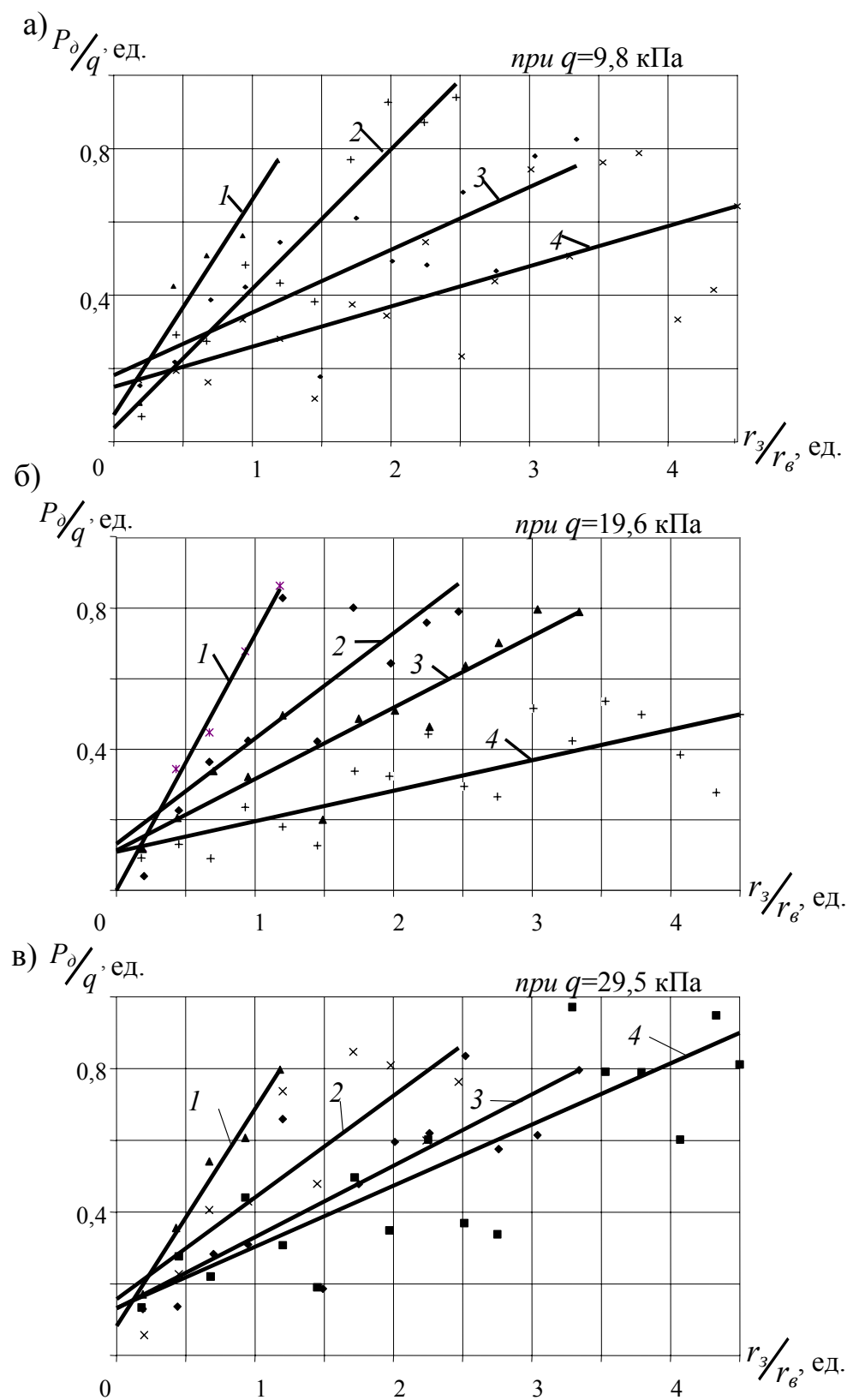
Рис. 3. Графики изменения вертикального давления P_d в пределах ЗПИ на уровне почвы выработки при различных значениях внешней пригрузки q и радиуса зоны r_3 (1, 2, 3, 4 – соответственно при радиусе ЗПИ: 1,2; 2,5; 3,4; 4,6 r_0 )
