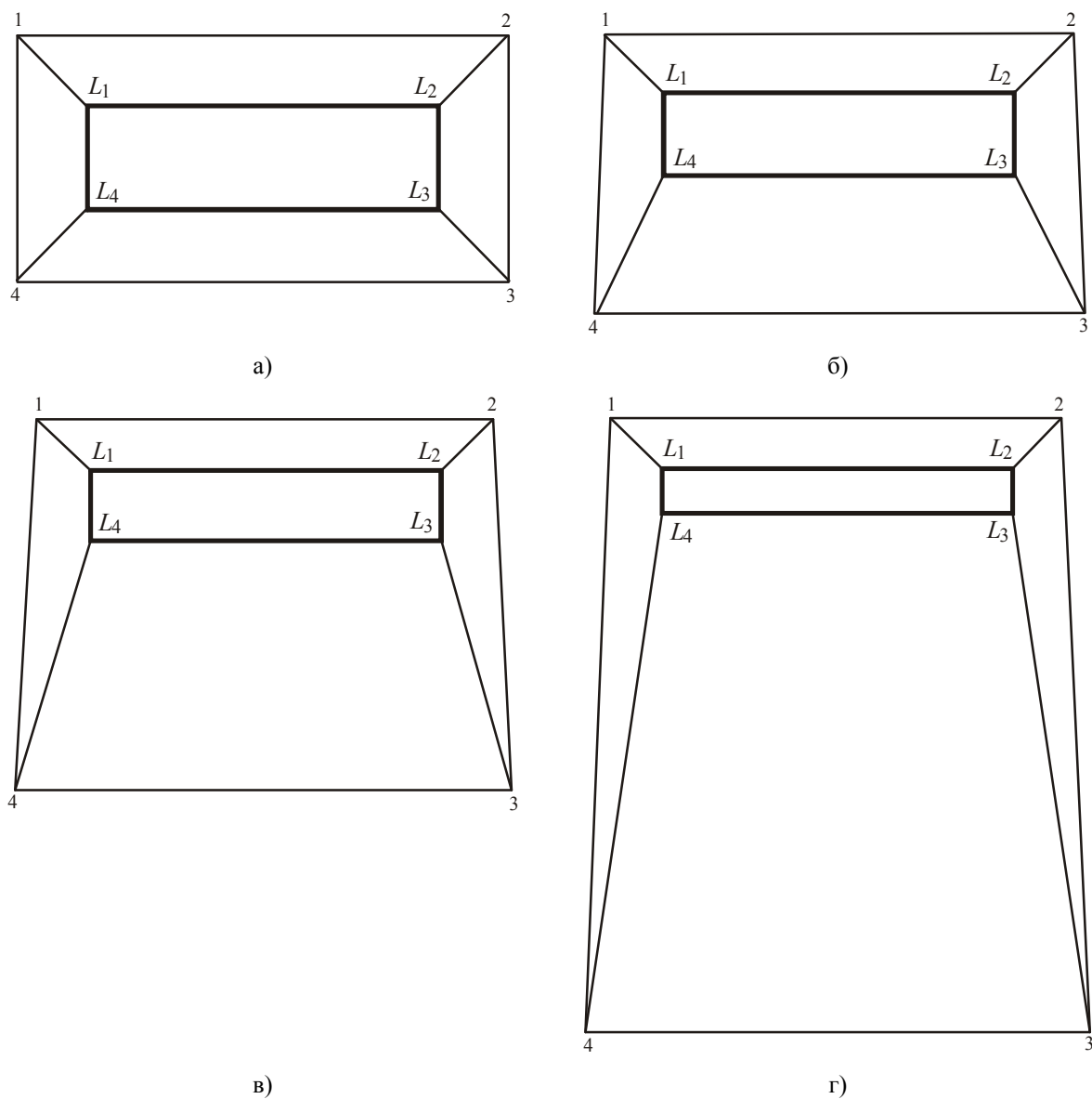
Рис. 3. Изменение формы мульды сдвижения с углом падения пласта: а) \alpha = 0^\circ ; б) \alpha = 20^\circ ; в) \alpha = 40^\circ ; г) \alpha = 60^\circ
