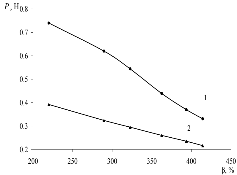
Рис. 4. Прочности алмазов ( P, H ) от содержания включений ( \beta, \% ) образцов № 1, № 3 и № 6: 1 – до термообработки (исх.); 2 – после термообработки
