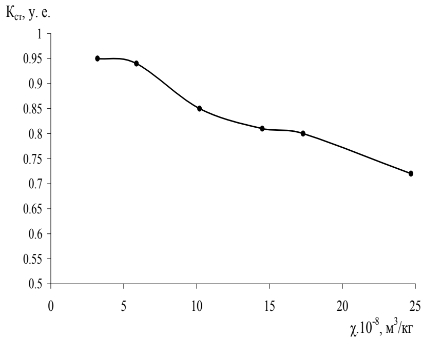
Рис. 2. Коэффициент термостабильности K_{ст} от удельной магнитной восприимчивости \chi
