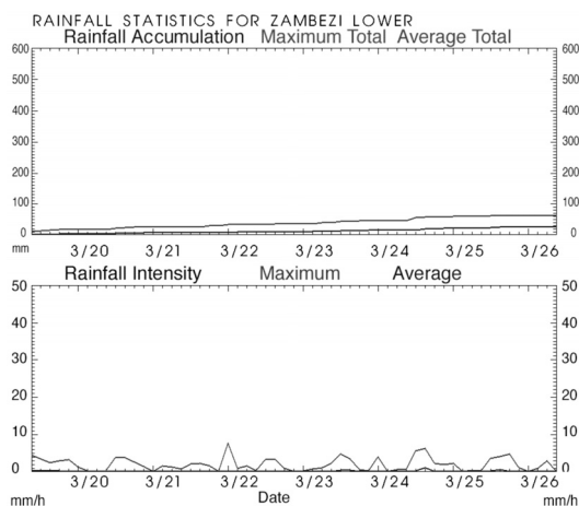
Рисунок 8 – Измерения уровня осадков
