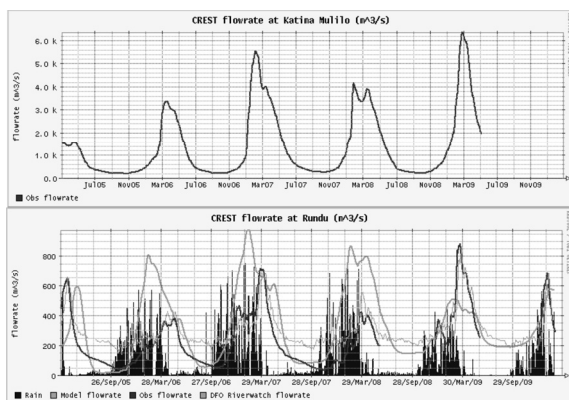
Рисунок 9 – Наземные измерения стока
