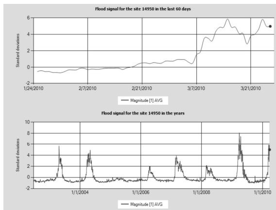
Рисунок 11 – Изменение уровня затоплений на разных временных интервалах
