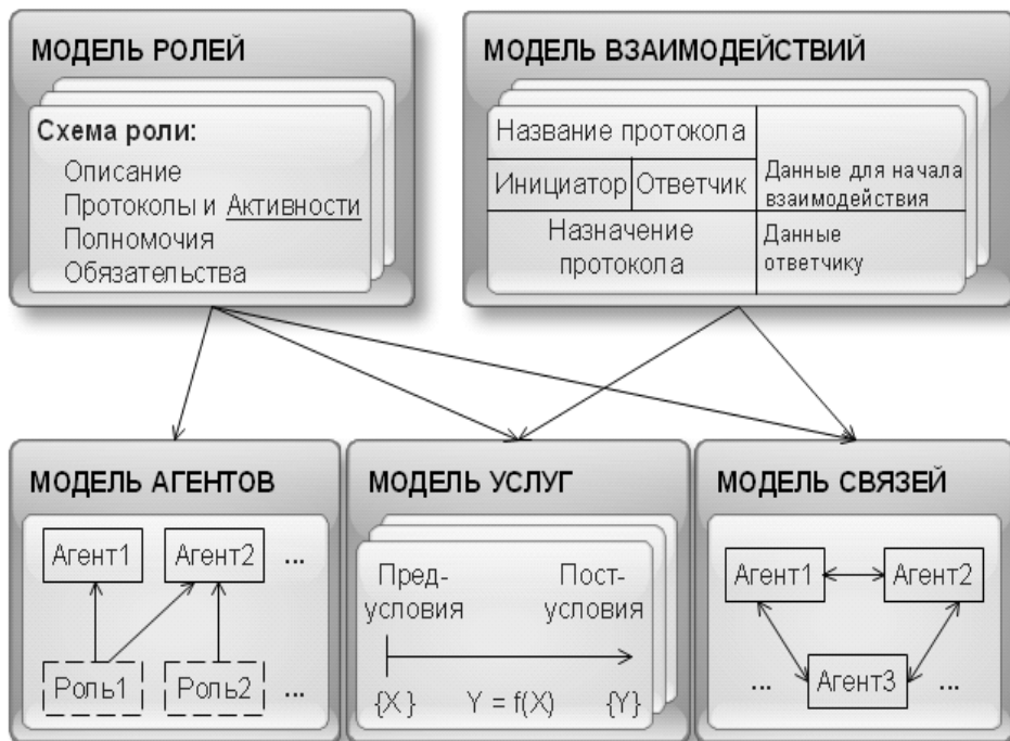
Рисунок 6 – Взаимосвязь абстрактных моделей при агентно-ориентированном проектировании по методологии Gaia
