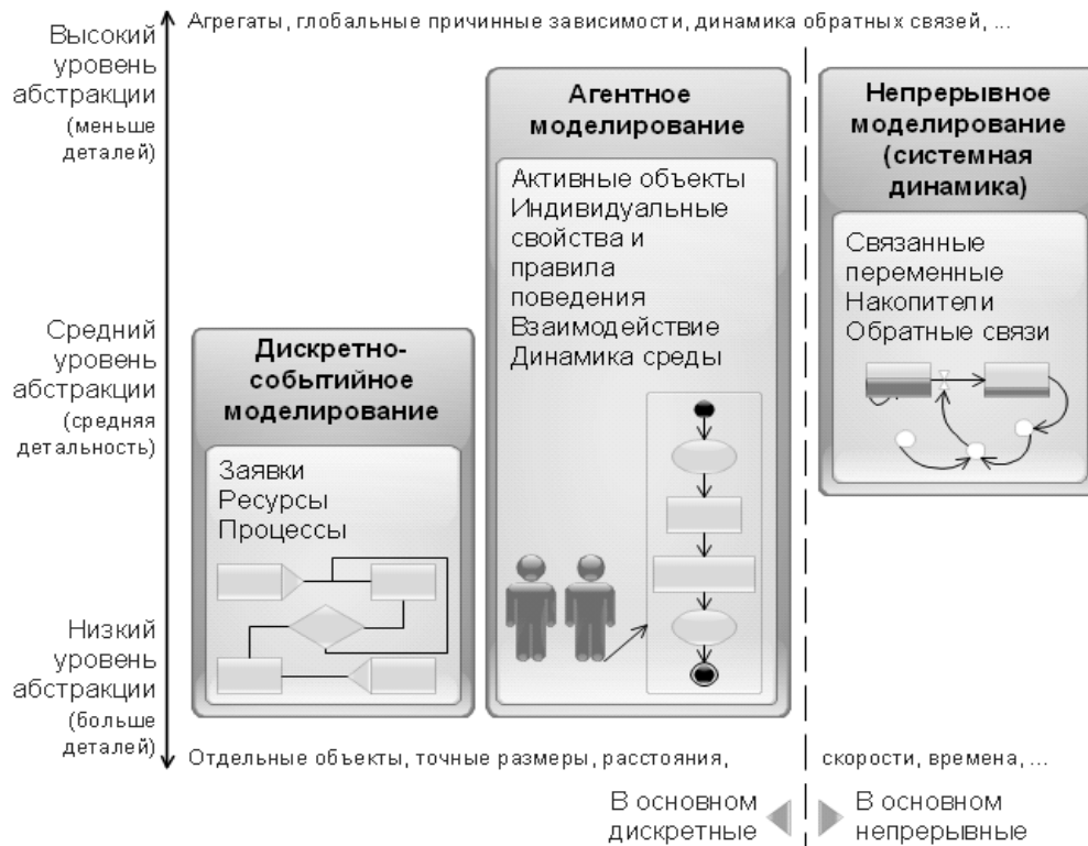
Рисунок 1 – Виды имитационного моделирования по уровню абстракции
