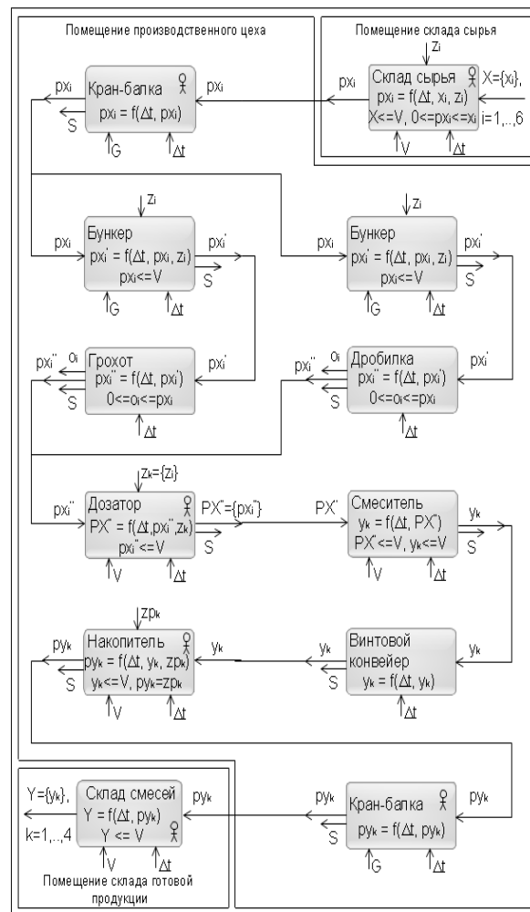
Рисунок 4 – Параметрическое описание автономных процессов при производстве промышленных смесей: x_i – запасы сырья i -ого типа, px_i – порция сырья i -ого типа, y_k – запасы смеси k -ого типа, py_k – порция смеси k -ого типа, z_i – количество требуемого сырья i -ого типа, z_k – количество требуемого сырья для приготовления смеси k -ого типа, V – вместительность/емкость, G – грузоподъемность, \Delta t – длительность технологической операции
