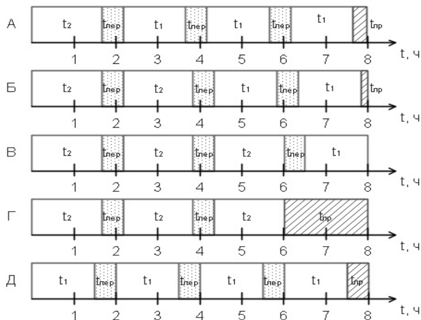
Рисунок 9 – Варианты технологических карт приготовления смесей в течение рабочего дня
