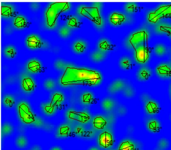
Рисунок 4 – Результат работы метода определения угла наклона выделенных областей изображения к горизонтальной оси
