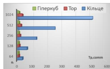
Рисунок 2 – Трудомісткість операцій обміну для LER-алгоритму з рівномірним способом розбиття від числа процесорів при складних правих частинах СЗДР для h^2 -екстраполяції
