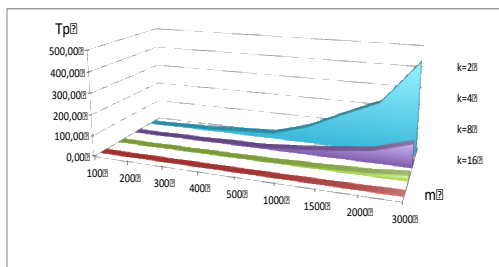
Рисунок 6 – Час паралельних обчислень за ЛЕР від розміру СЗДР для регулярного розбиття при p = 32 для різної довжини ET ( \mu s )
