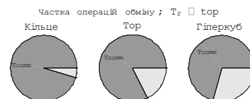
Рисунок 1 – Частка операцій обміну до загальних накладних витрат для LER-алгоритму з пропорційним способом розбиття при тривіальних правих частинах СЗДР для h^2 -екстраполяції
