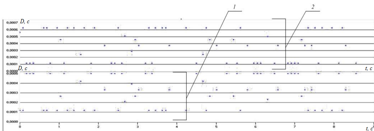
Рисунок 8 – Діаграма затримки між роутером і коммутатором А: 1 – від роутера до коммутатора А; 2 – від коммутатора А до роутера
