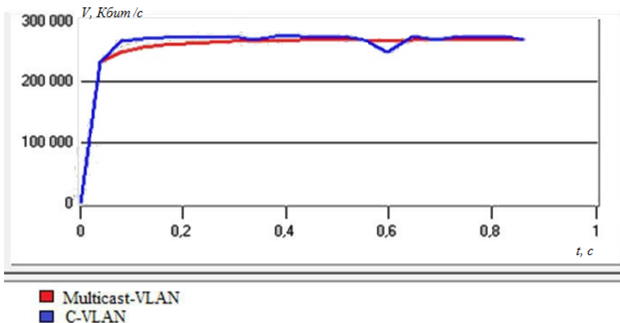
Рисунок 4 – Результаты моделирования различных схем VLAN
