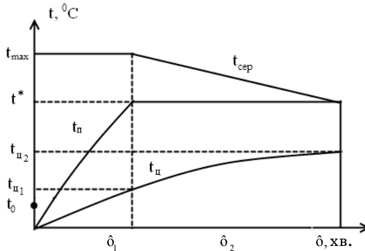
Рис. 1. Зміна температури нагрівного середовища і продукту в процесі 2-х стадійної термообробки:
