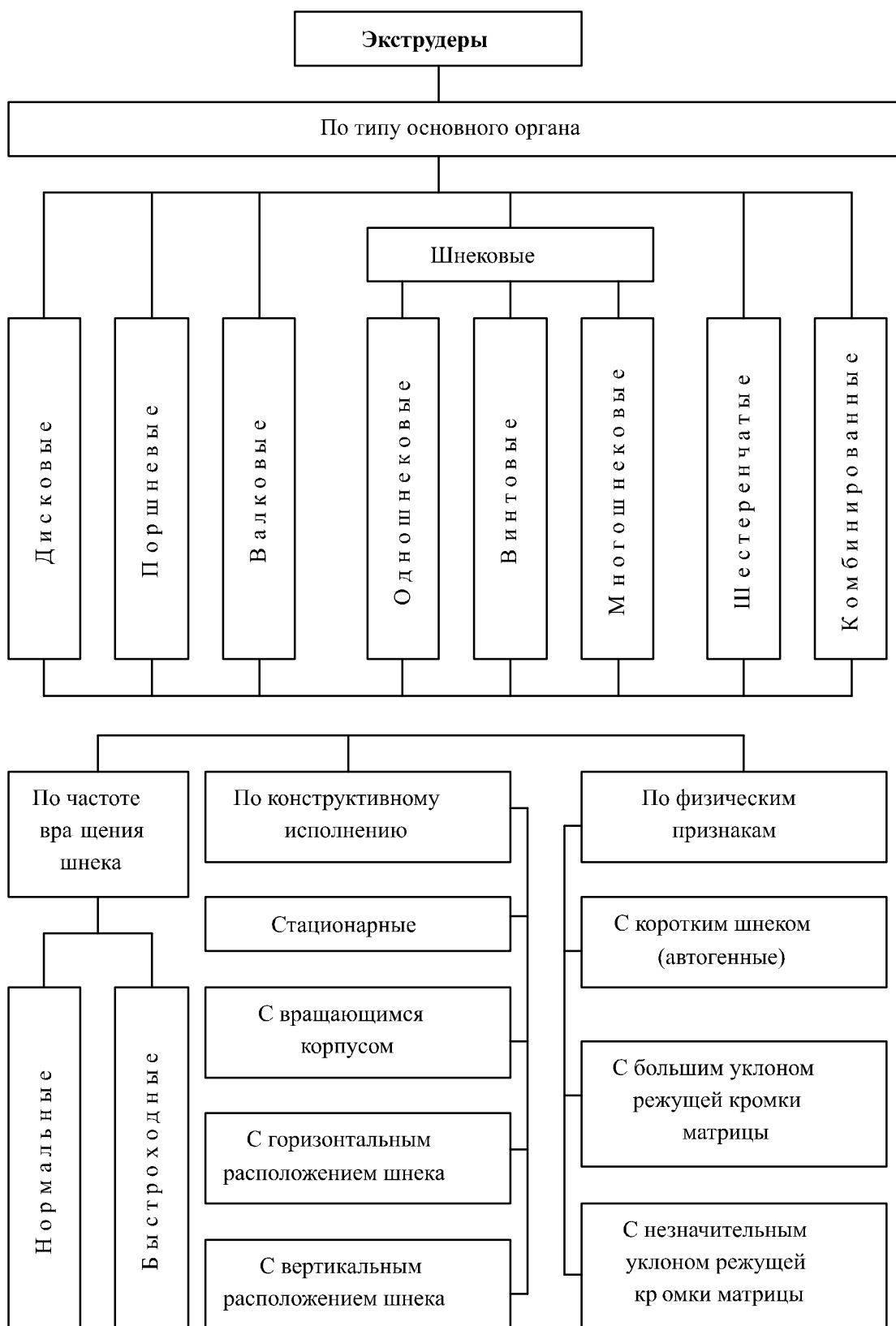
Рис. 1. Классификация экструдеров
