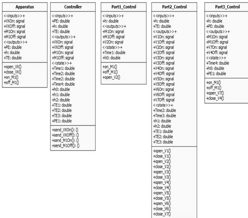
Рис. 2. Діаграма класів
