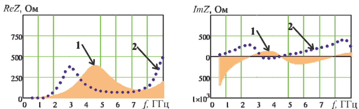
Рисунок 2 – Входной импеданс щелевого и дипольного излучателей: 1 – диполь в свободном пространстве; 2 – одиночная щель в экране
