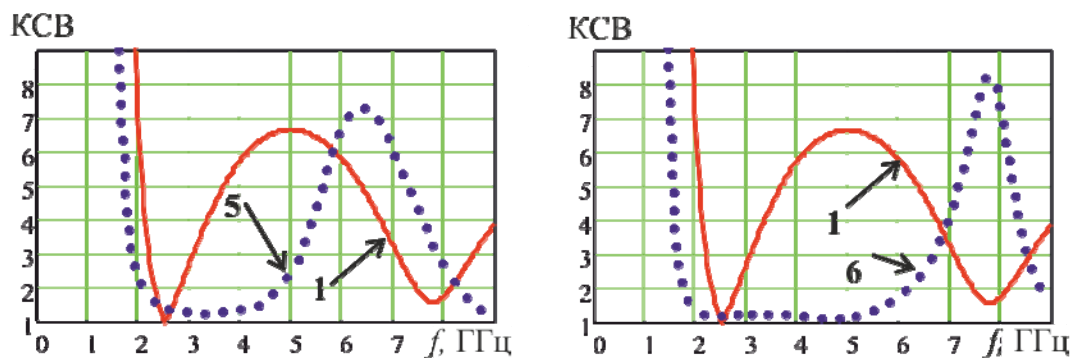
Рисунок 10 – Частотные зависимости КСВ дискретно-щелевых антенн: 5 – двухщелевая антенна, 6 – четырехщелевая антенна
