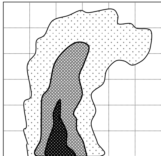
Рисунок 7 – Концентрация радиоактивного аэрозоля 15 июля 1990 г. ( \bar{D}_1 = 2,37 \cdot 10^{-9} \text{ Еи л}^{-3} , \bar{D}_2 = 1,25 \cdot 10^{-8} \text{ Еи л}^{-3} , \bar{D}_3 = 2,39 \cdot 10^{-8} \text{ Еи л}^{-3} в 24^{00} - 24^{10} , 3-я труба)
