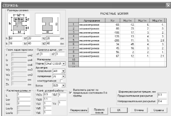
Рис.6. Общий вид программы «Сечения железобетонных элементов»
