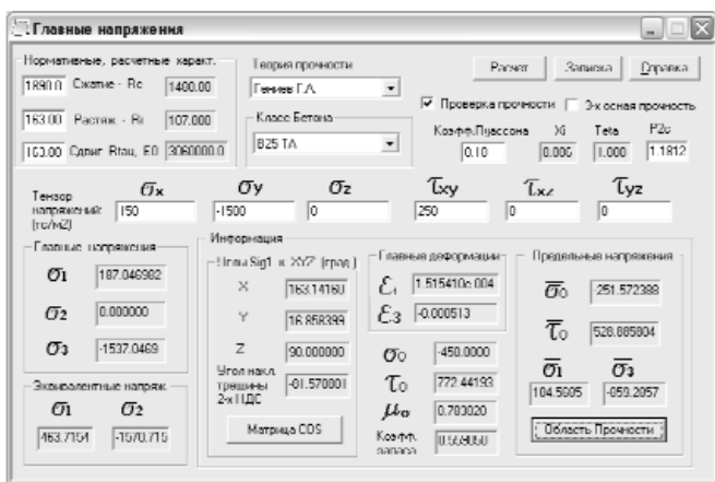
Рис.7. Общий вид программы «Главные и эквивалентные напряжения»
