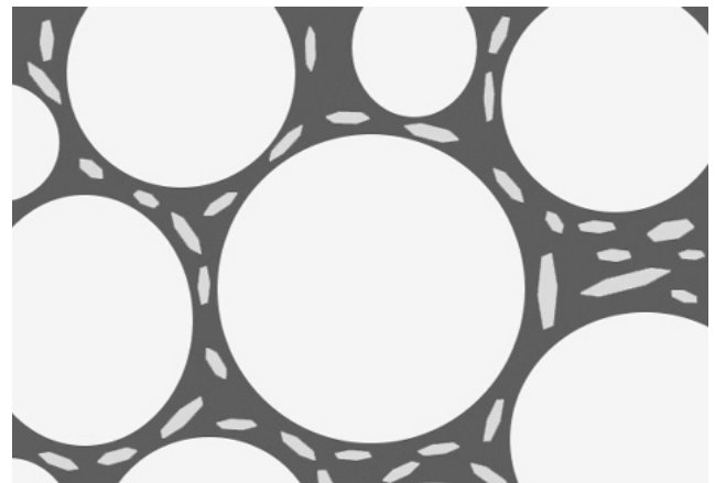
Рис. 2. Схематическое изображение структуры пенобетона: круглыми белыми кругами обозначены поры; черным — цементный раствор; серым — частицы шлама
