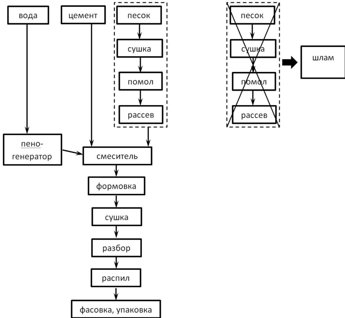
Рис. 4. Общая технологическая схема производства блоков пенобетона
