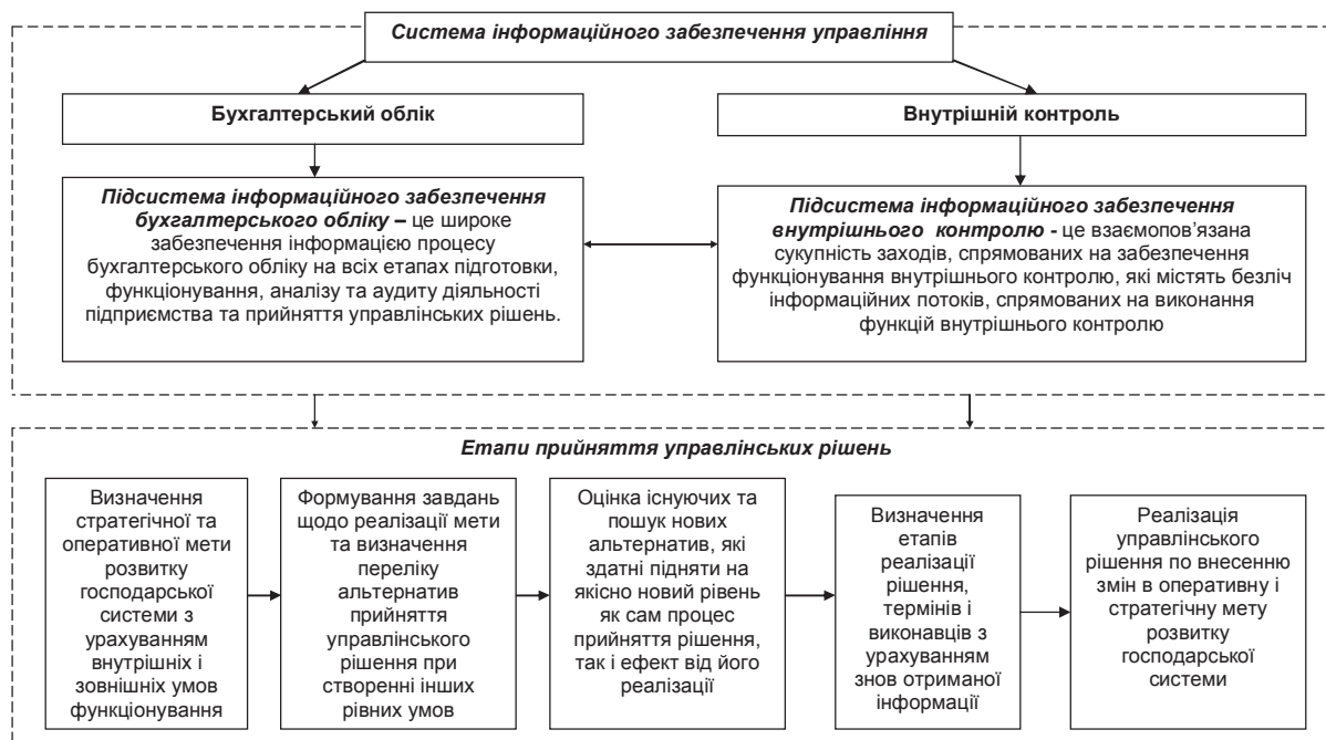
Рис. 2. Облік та внутрішній контроль у формуванні інформаційного забезпечення управління підприємством
