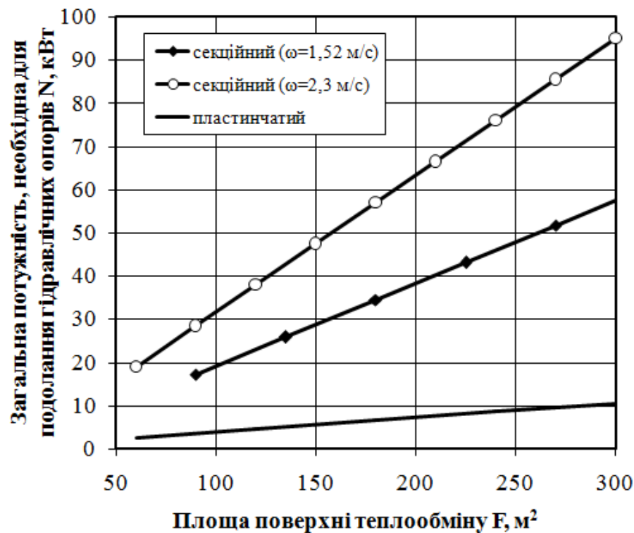
Рис.2. Залежність загальної потужності, необхідної для подолання гідравлічних опорів, від площі поверхні теплообміну
