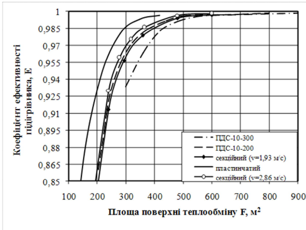
Рис.3. Залежність коефіцієнта ефективності групи нагріву підігрівників від площі поверхні теплообміну
