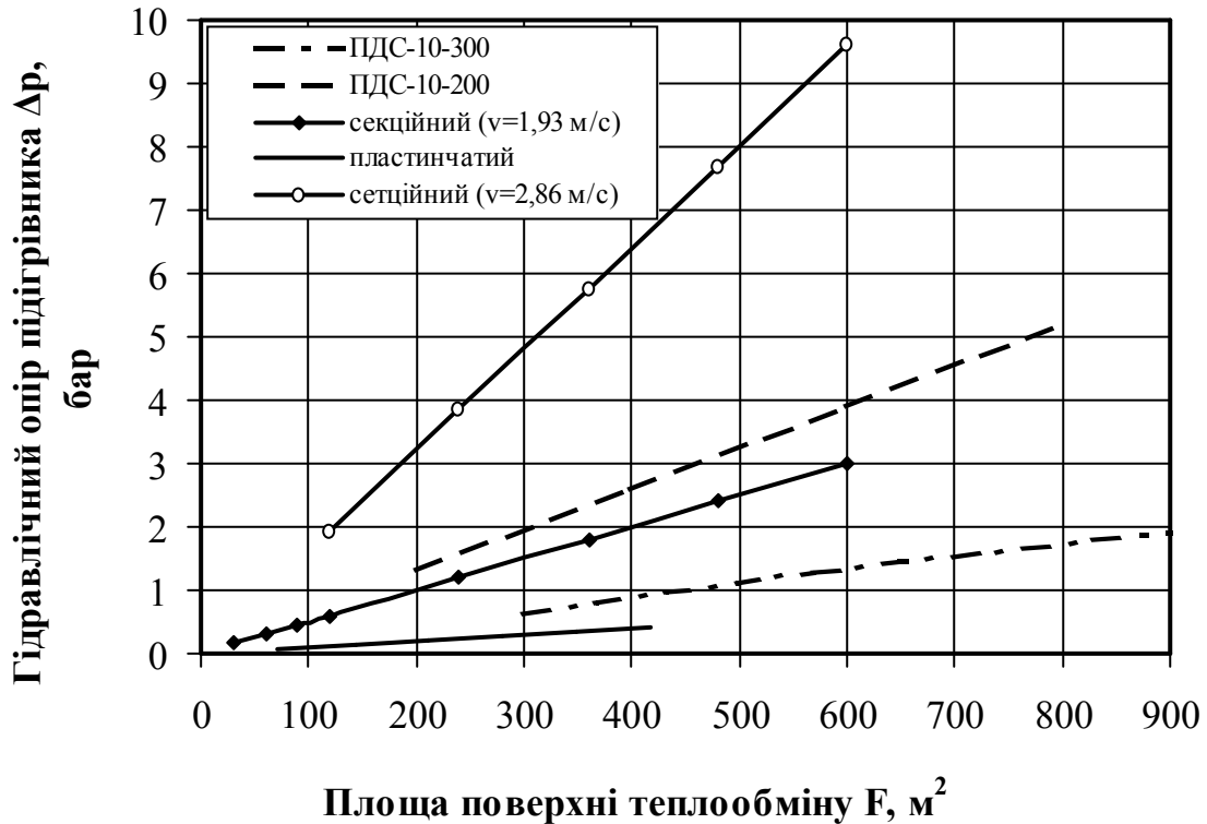
Рис.4. Залежність гідравлічного опору групи нагріву підігрівників від площі поверхні теплообміну
