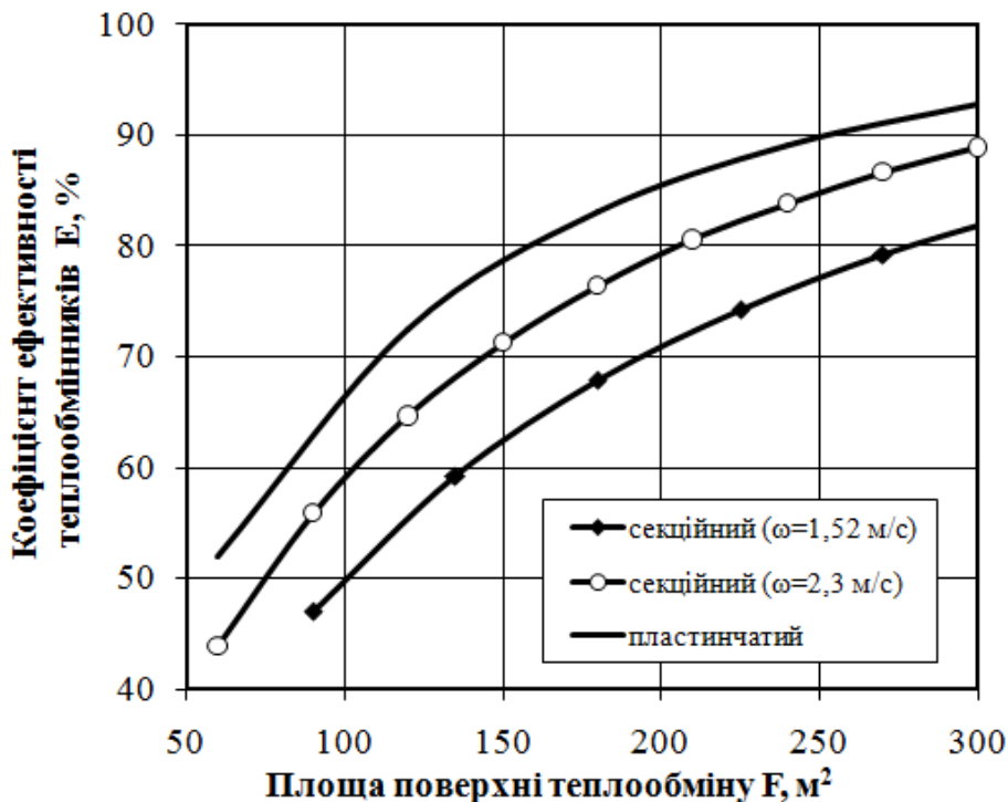
Рис.1. Залежність коефіцієнта ефективності групи нагріву теплообмінників від площі поверхні теплообміну
