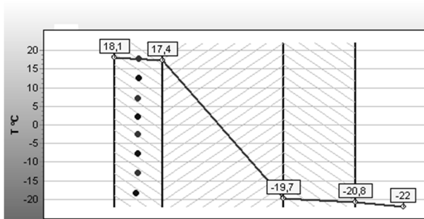
Рис. 5 Теплопотери в плоскости компенсационной системы наружной стены.
