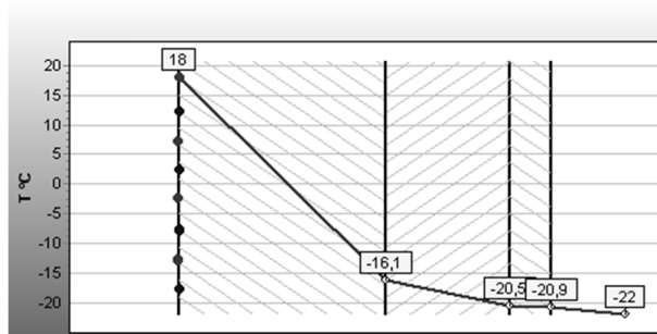
Рис. 6 Теплопотери в плоскости компенсационной системы от кровельной части.
