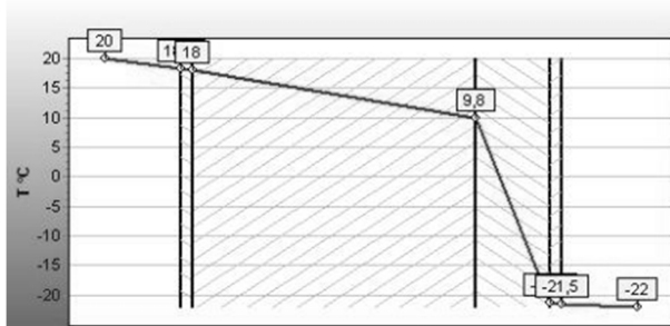
Рис. 1 График температуры внутри многослойной конструкции 0,51 м (0,015 м штукатурка, 0,38 м кирпичная кладка, 0,10 м теплоизоляции, 0,015 м штукатурка)
