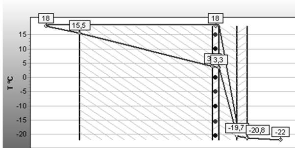
Рис.4 Температурный режим в плоскости компенсационной системы наружной стены с учётом теплоносителя
