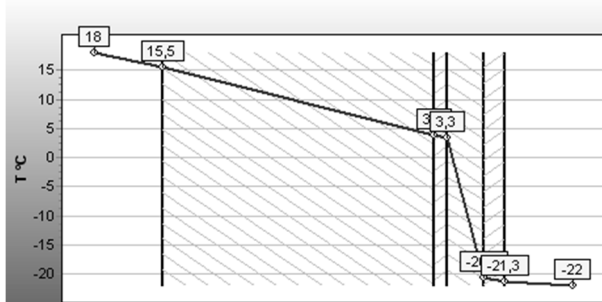
Рис. 3 Температурный режим в плоскости компенсационной системы наружной стены.
