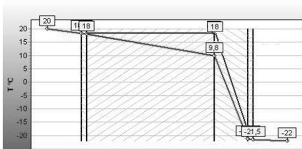
Рис. 2 График температуры внутри многослойной конструкции с учётом размещения настенного компенсатора.
