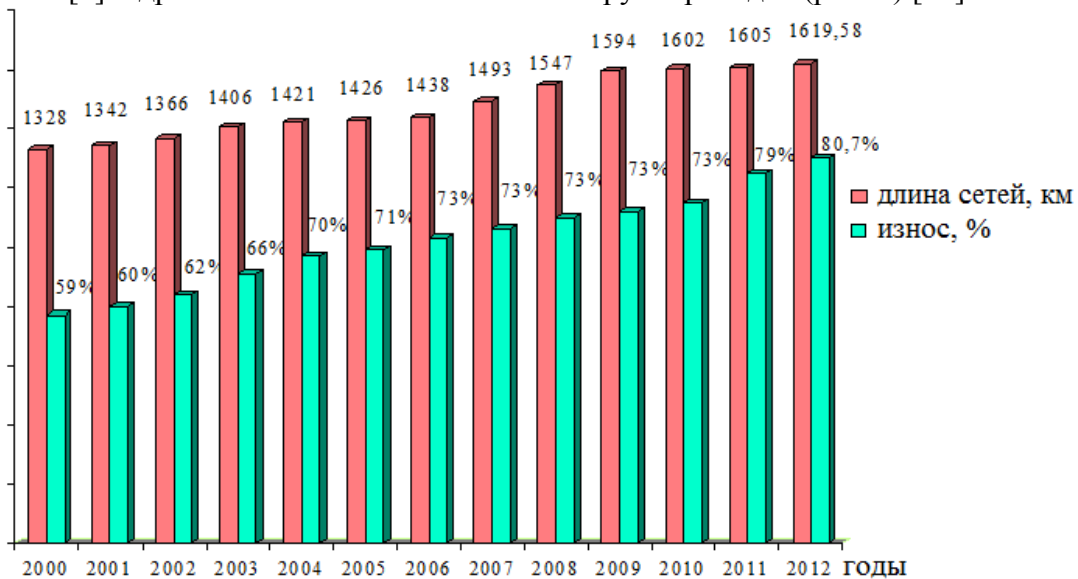
Рис. 1. Длина канализационных сетей Харькова по состоянию на 01.01.2012 г.
