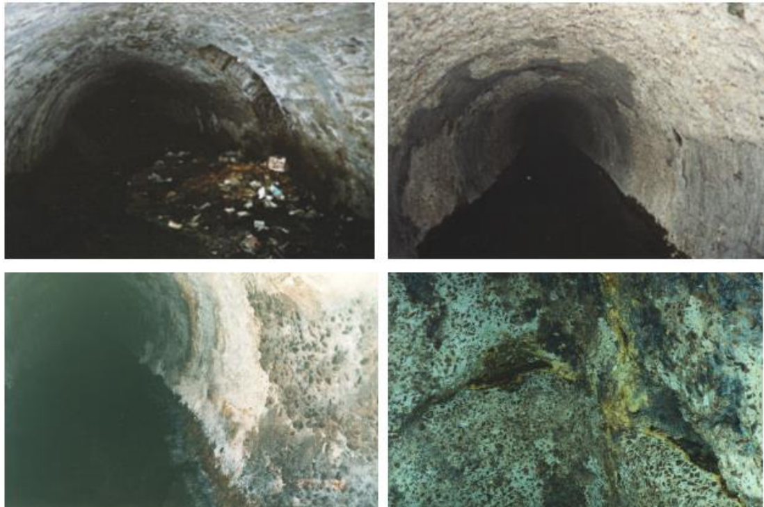
Рис. 4. Внутренняя поверхность канализационных тоннельных коллекторов, разрушенная внутренней коррозией
