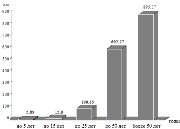
Рис. 3. Характеристика канализационных сетей за показателем срока эксплуатации
