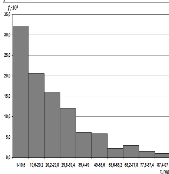
Рис. 1. Гістограма розподілу часу відновлення працездатності t_i
