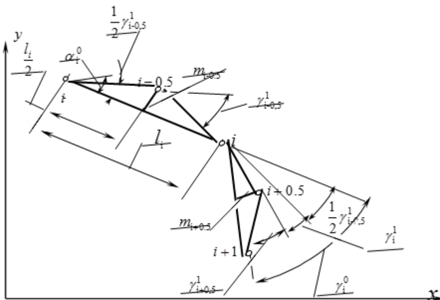
Рис.2. Фрагмент, построенный с помощью серединных перпендикуляров
