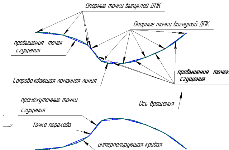
Рис. 1. Схема построения устройства с переменным живым сечением, внутренняя поверхность которого построена методом серединных перпендикуляров
