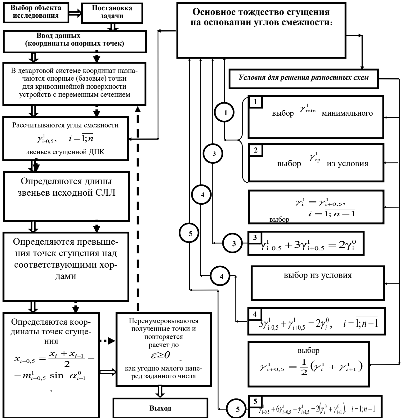
Рис. 3. Алгоритм расчёта процесса построения криволинейной внутренней поверхности с изменяющимся живым сечением с помощью серединных перпендикуляров:
