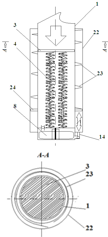
Рис. 5. Схема розташування пневмомеханічної муфти акумуляції (у подовжньому та поперечному розрізі) 1 – корпус; 3 – дно-поршень; 4 – центральна пружина; 8 – лопать турбіни; 14 – пневмотруба; 22 - пневмомеханічна муфта акумуляції; 23 - циліндрова пружина; 24 – кільцевий поршень
