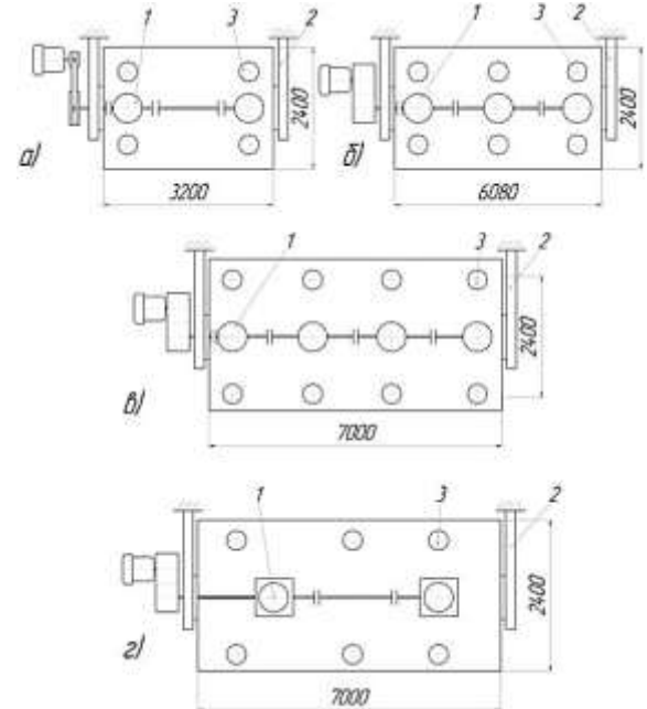
Рис. 1. Конструктивні схеми ударно-струшуючих установок
