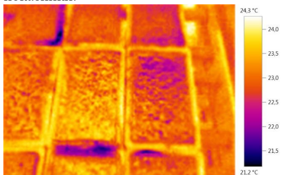
Рис. 5. Розподіл температури всередині камери після відкриття кришки (фрагмент № 2)
