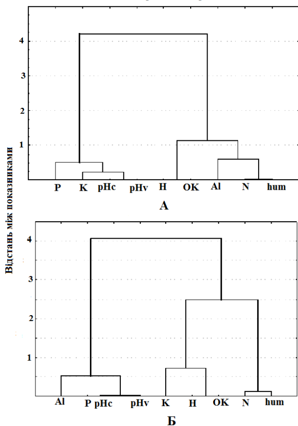
Рис. 3. Дерево зв'язків між показниками ґрунтів лучних (А) та лісових (Б) екотопів.
