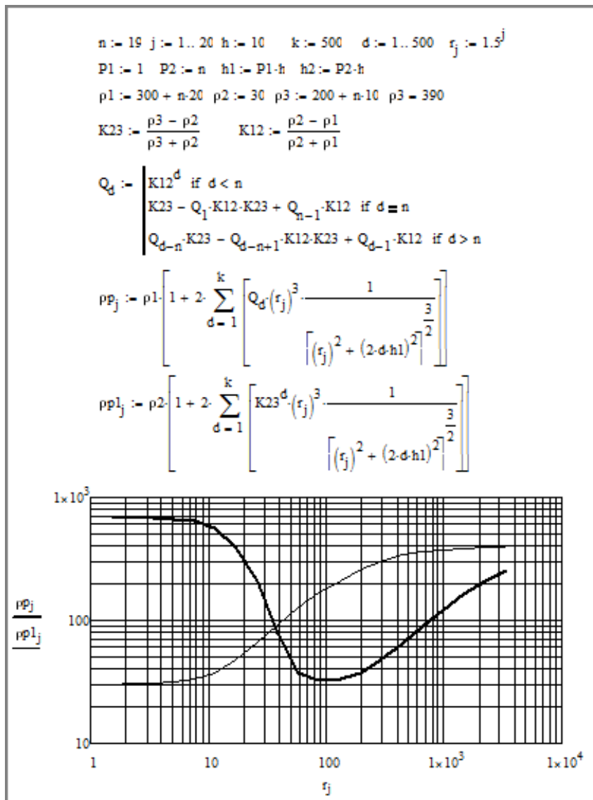
Рисунок 2 – MathCAD-документ розв’язання прямої задачі вертикальних електричних зондувань
