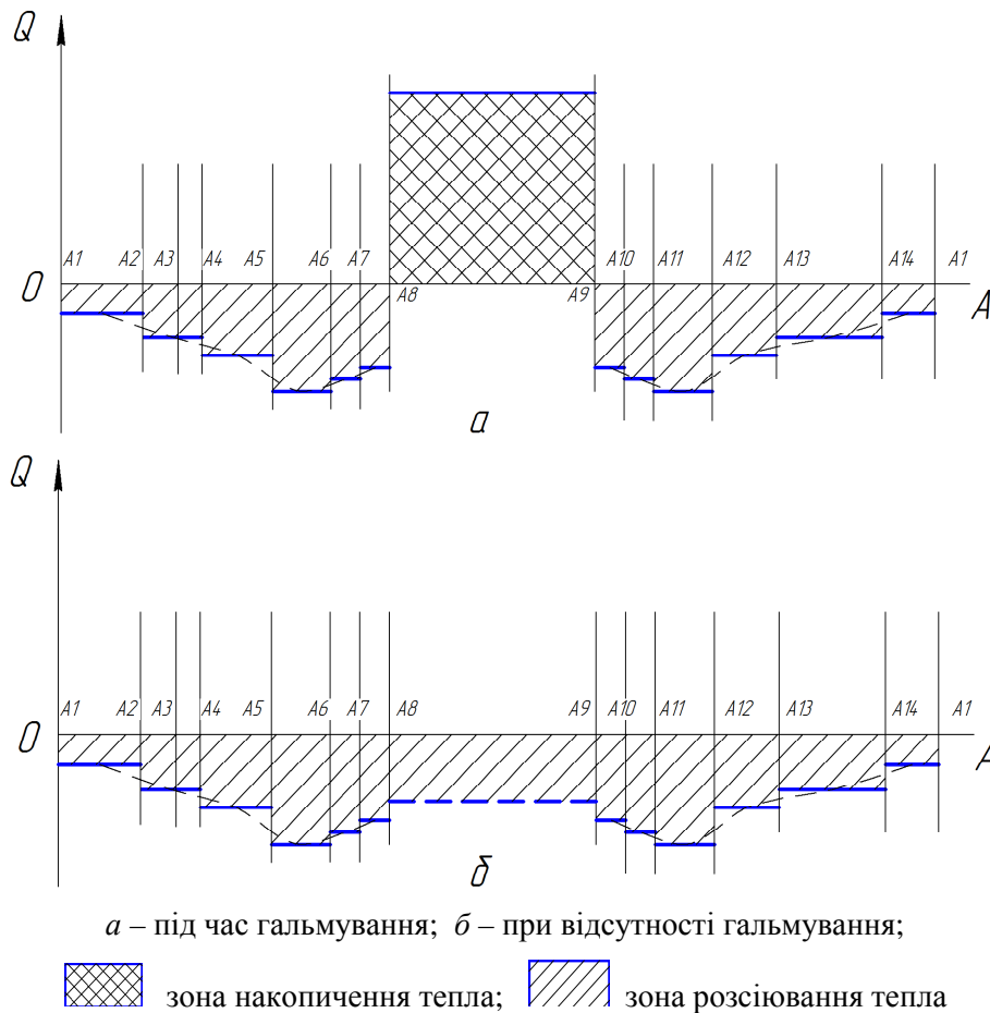
Рисунок 2 – Графіки теплових потоків поверхонь шків стрічково-колодкового гальма
