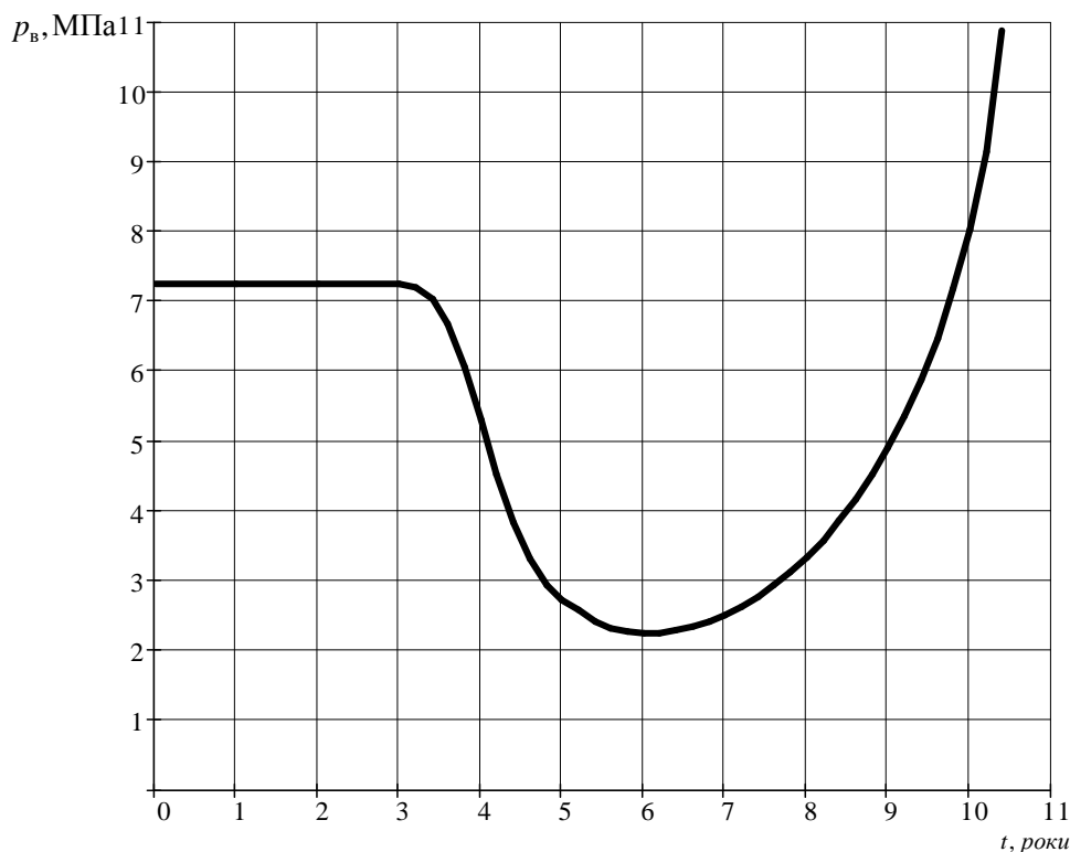
Рисунок 4 – Зміна вибійного тиску p_v фонтанування в часі t
