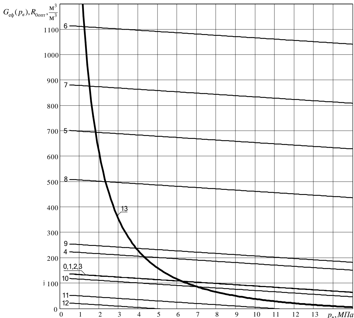
Рисунок 3 – Визначення мінімального вибійного тиску p_b(t) на момент часу t , роки: 0,1,2,3 лінії (0,1,2,3); 4(4); 5(5); 6(6); 7(7); 8(8); 9(9); 10(10); 11(11);12(12), залежно від змінного тиску p_b для заданої функції питомі витрати газу R_0(t) (лінія 13)
