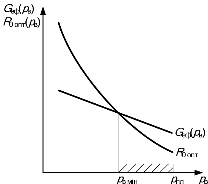
Рисунок 1 – Графічна інтерпретація умови газліфтного фонтанування свердловини (область можливого фонтанування заштриховано між тисками пластовим \rho_{пл} і мінімальним вибійним \rho_{в\ мін} )
