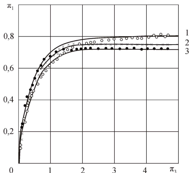
Рисунок 1 – Кінетика намивання шару дисперсної фази в тріщині за різних значень параметра \pi_2 : 657 (1); 922 (2); 1078 (3)
