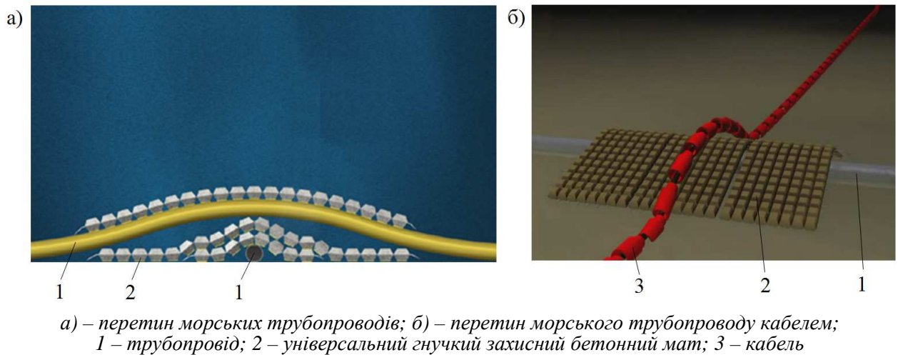
Рисунок 7 – Застосування універсальних гнучких захисних бетонних матів у місці перетину морських трубопроводів та кабелів
