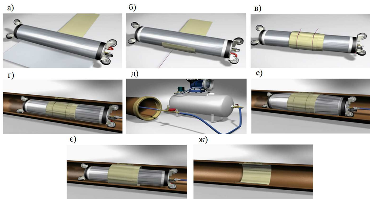
а) – намотування фольги; б) – намотування композитного бандажу; в) – закріплення бандажу; г) – доставляння пристрою до місця ремонту; д) – нагнітання повітря в пристрій; е) – розширення пристрою; є) – стравлювання повітря з пристрою; ж) – підсилений бандажем трубопровід
