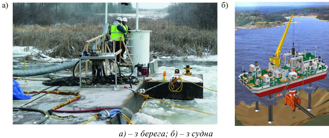
Рисунок 12 – Встановлена підводна камера з шахтним колодязем
