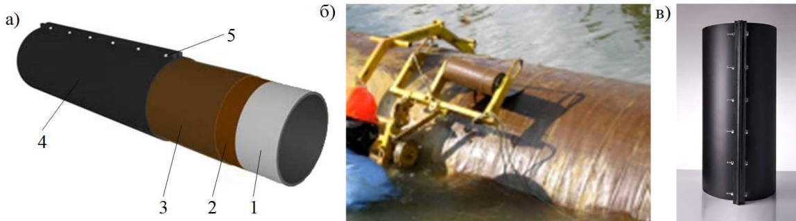
а) – конструкція ізоляції; б) – нанесення петролатумної стрічки намотувальним верстатом; в) – захисний кожух; 1 – трубопровід; 2 – ґрунтовка; 3 – петролатумна стрічка; 4 – захисний кожух; 5 – болтове з'єднання
