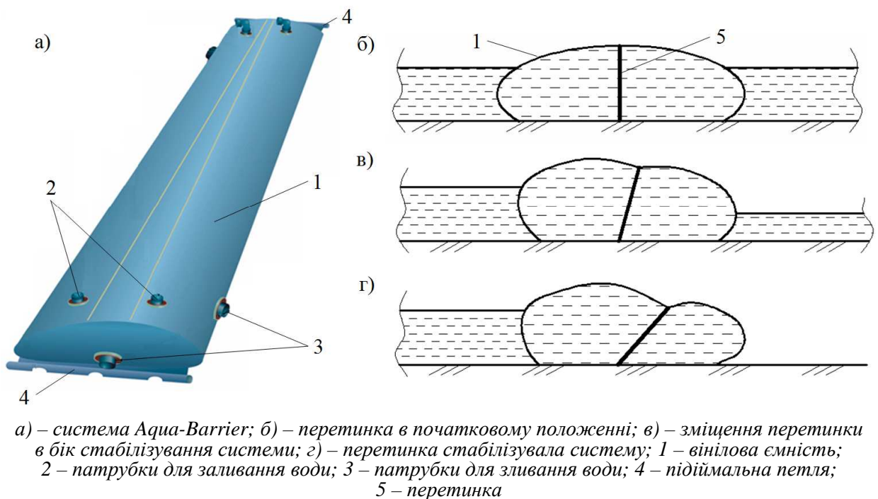
Рисунок 8 – Принцип роботи системи Aqua-Barrier
