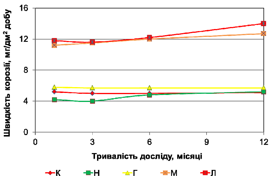
Рисунок 2 – Зміна швидкості корозії сталевих зразків в довготривалому експерименті
