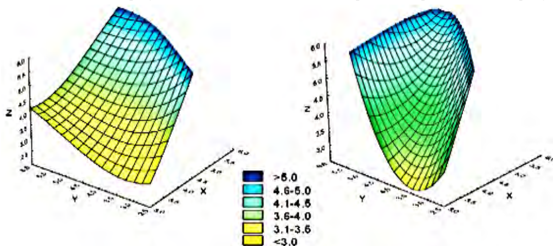
Рис. 1. Варіювання вмісту гумусу згідно з даними різних інтерполяторів:
