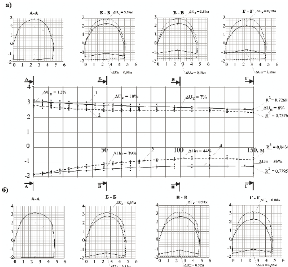
Рис. 5. Графики смещения пород кровли (1,2) и почвы (3,4) на контрольном (1,3) и экспериментальном (2,4) участках: \Delta U_{п} – разность смещений на контрольном и экспериментальном участках, %
