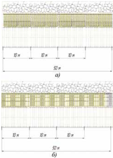
Рис. 4. Схема расположения замерных станций на контрольном (а) и экспериментальном (б) участках
