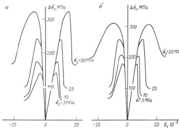
Рис. 2. Зависимости напряжений \Delta\sigma_1 от деформации \epsilon_1 и \epsilon_2 для выбросоопасного (а) и невыбросоопасного (б) песчаников при разных уровнях гидростатического давления \sigma_2 по данным А.Н. Ставрогина
