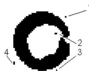
Рис. 2. Корректировка контура капли воды в масле: 1–4 – шумы
