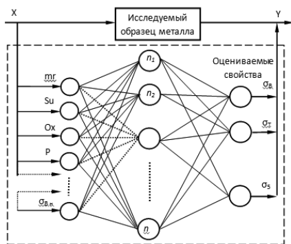
Рис. 5. Нейронная сеть оценки свойств металла
