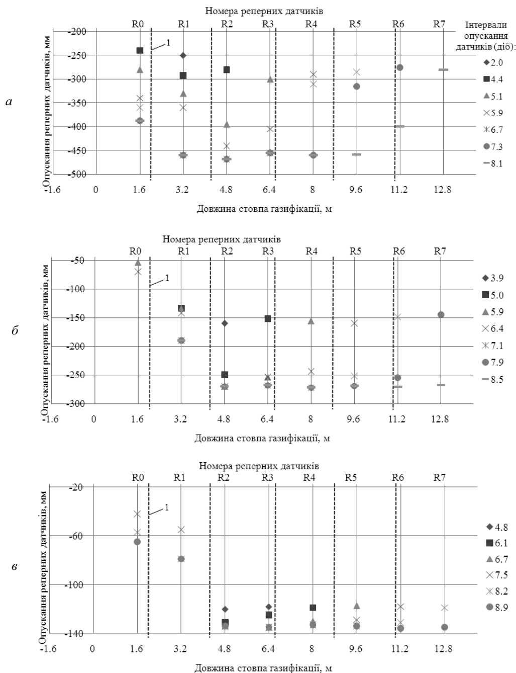
Рис. 2. Мережа усереднених значень опускань порід підовши верхнього вугільного пласта при потужності міжпластових порід 3,6 (а), 5,4 (б) та 6,6м (в) за замірними точками: 1 – розташування вогневого вибою (посування 2,2м/добу)
