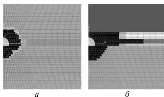
Рис. 3. Конфигурация техногенной газовой залежи вокруг одиночной полости, заложеной в однородном (а) и слоистом (б) массивах
