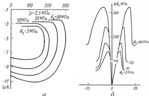
Рис. 1. Изменение газовой проницаемости k (а) образцов песчаника на разных этапах их деформирования (б) по данным Ставрогина А.Н., Протосени А.Г., где \sigma_2 = \sigma_3 – боковая нагрузка; \Delta \sigma_1 – превышение осевой нагрузки \sigma_1 над боковой
