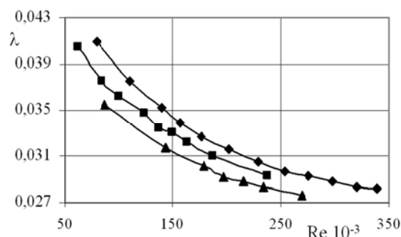
Рис. 2 Зависимость \lambda от Re при разных \mu_{\text{мас}}/\mu_1 : \blacklozenge – n=1 (изотермическое течение); \blacksquare – n=0,65 ; \blacktriangle – n=0,45
