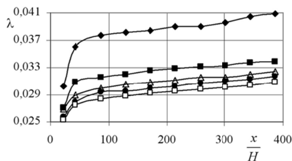
Рис. 1 Изменение гидравлического коэффициента трения вдоль канала: \blacklozenge – v_0 = 5 \text{ м/с} ; \blacksquare – v_0 = 10 \text{ м/с} ; \triangle – v_0 = 12 \text{ м/с} ; \bullet – v_0 = 13 \text{ м/с} ; \square – v_0 = 15 \text{ м/с}
