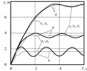
Рис. 2. Графические зависимости движения под- весной монорельсовой дороги во времени: а – T_{q1}(t) = 30\text{ кН}; T_{q9}(t) = 0 ; б – T_{q1}(t) = T_{q9}(t) = 30\text{ кН} ; в – T_{q1}(t) = T_{q9}(t) = Fq_2(t) = Fq_8(t) = 30\text{ кН}
