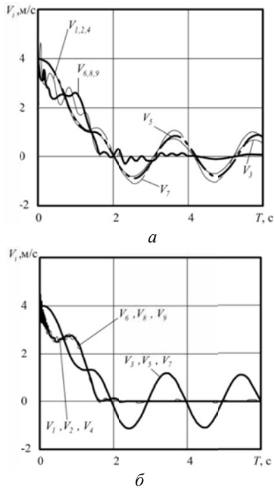
Рис. 3. Зависимости изменения скорости движения подвесной монорельсовой дороги во время торможения при: а - c_c = 800 кН/м; б - c_c = 8000 кН/м
