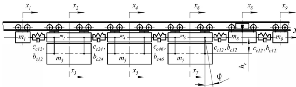
Рис. 1. Расчетная схема продольных колебаний подвижного состава
