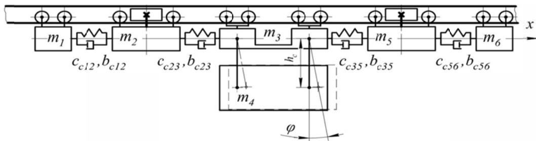
Рис. 4. Расчетная схема продольных колебаний крупногабаритного груза, перевозимого подвесной монорельсовой дорогой
