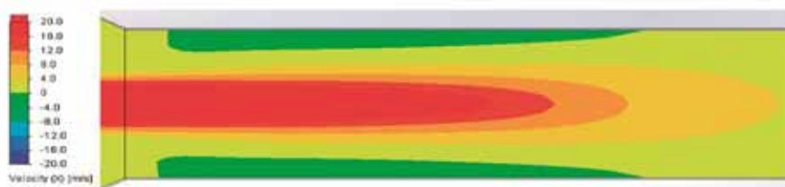
Рис. 1. Ізолінії поздовжньої проекції швидкості рідини в камері змішування центрального ежектора ( m = 11 ; q = 0,5 )
