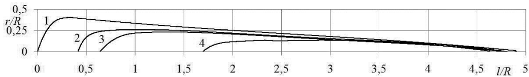
Рис. 2. Геометричні параметри ТЗ для центрального ежектора з m = 5 і коефіцієнтом ежекції q = 0,1 (1); q = 0,25 (2); q = 0,35 (3); q = 0,5 (4)
