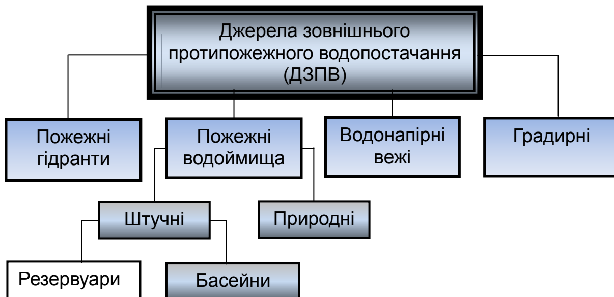
Рисунок 1 – Класифікація джерел зовнішнього протипожежного водопостачання
