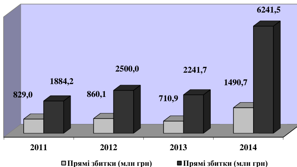
Рисунок 2 – Динаміка зміни прямих і побічних збитків від пожеж за 2011÷2014 роки
