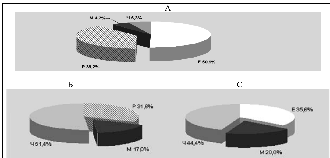
Рис. 2. Соотношение видового разнообразия Соперода в изучаемых районах: А- акватория Севастопольской бухты, 131 вид, Б- в эстуарной зоне Севастопольской бухты, 35 видов, С- в низовье русла реки Черная, 46 видов Fig.2. Ratio of copepoda species diversity: А – in Sevastopol Bay, 131 sp., Б- in estuarine zone, 35 sp., С- in of lower reach of Chernaya river, 46 sp.
