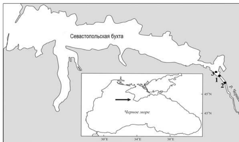
Рис. 1. Карта-схема станций отбора проб в районе исследования
