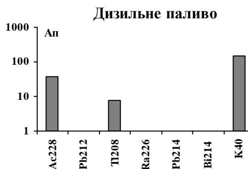
Рис.8. НСТ зразка «дизельне паливо». Ап , Бк/кг
