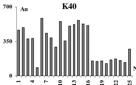
Рис.3. НСЗ K40. A_n , Бк/кг.
