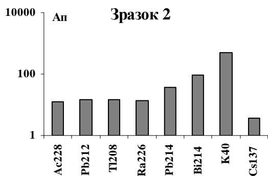
Рис.4. НСТ зразка «нафта №2». Ап , Бк/кг
