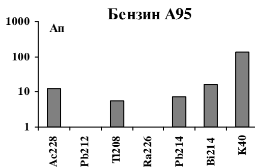
Рис.7. НСТ зразка «бензин А95». Ап , Бк/кг
