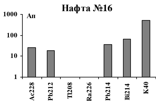
Рис.6. НСТ зразка «нафта №16». Ап , Бк/кг
