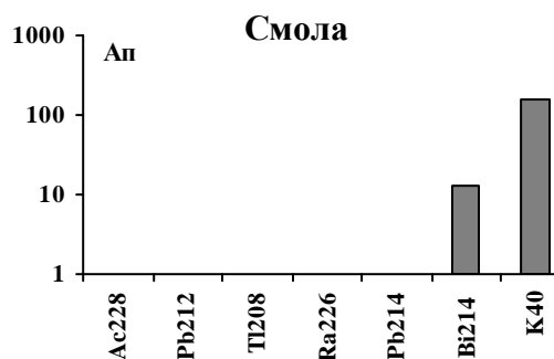
Рис.10. НСТ зразка «смола». Ап , Бк/кг
