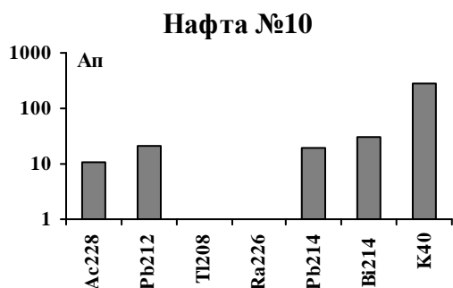
Рис.5. НСТ зразка «нафта №10». Ап , Бк/кг
