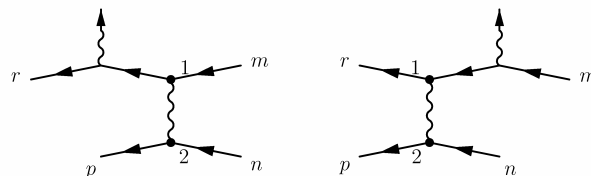
Рис. 1. Фейнманівські діаграми ефектів третього порядку КЕД.
