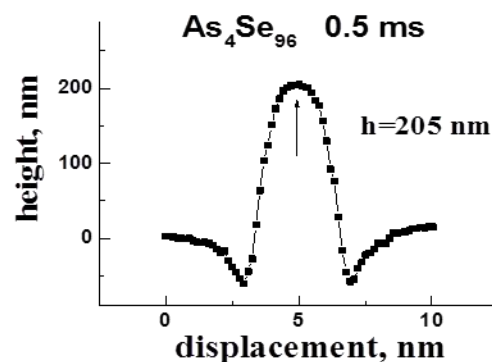
Рис.1. АСМ-зображення та профілі поверхневого рельєфу, індукованого електронним променем на поверхні плівки \text{As}_4\text{Se}_96 , які формуються в області доз 9.3 \times 10^2 мкКл/см 2 - 9.3 \times 10^3 мкКл/см 2 .
