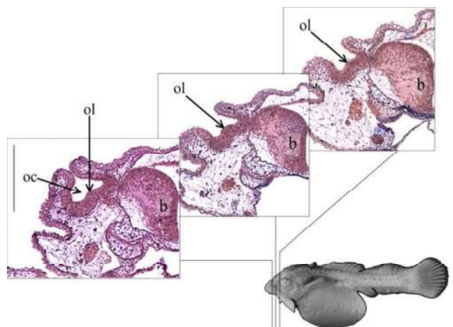
Рис. 1. Поперечний переріз через нюхову камеру A. dolichopterus (SL = 7 мм): ol – нюхова ламела; b – головний мозок, oc – нюхова порожнина. Scale bar = 200 \mu m.
