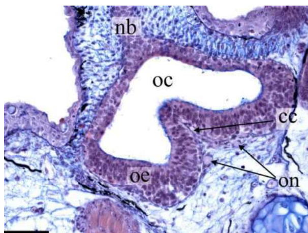
Рис. 2. Поперечний переріз через першу нюхову ламелу A. dolichopterus (SL = 8,5 мм):
