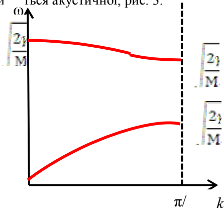
Рис. 3. Закон дисперсії коливань ланцюжка двоатомної системи
