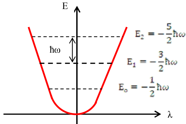
Рис. 4. Енергетичні рівні
