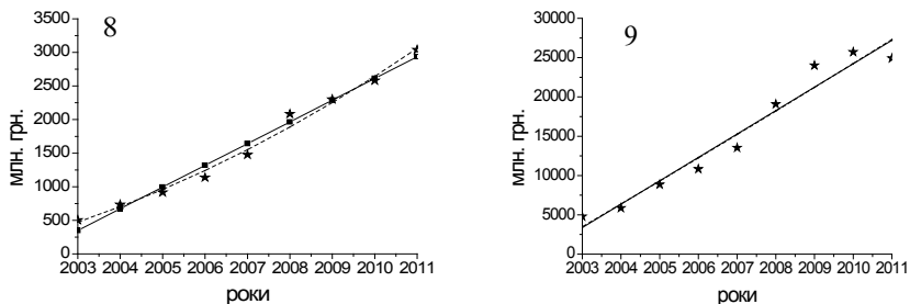
Рис. 3. Лінійні та квадратичні апроксимації розподілу за часом обсягів витратків споживання та їх вихідні значення за напрямками духовний/фізичний розвиток та освіта)
